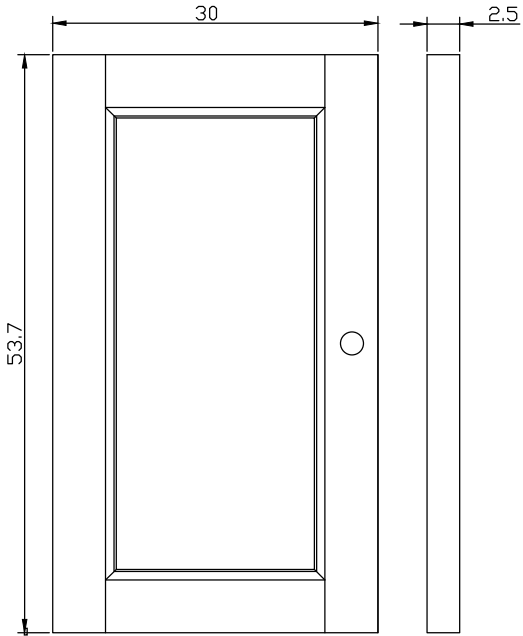
DETAIL DOOR
