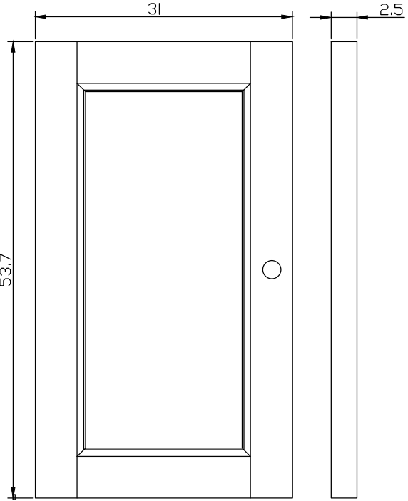
DETAIL DOOR
