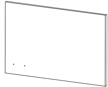
N01 Barbecue cabinet right door panel *1 360*580*16
