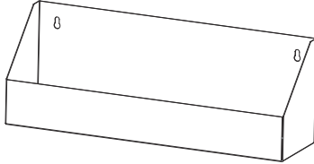
Container *2 460*120*165
