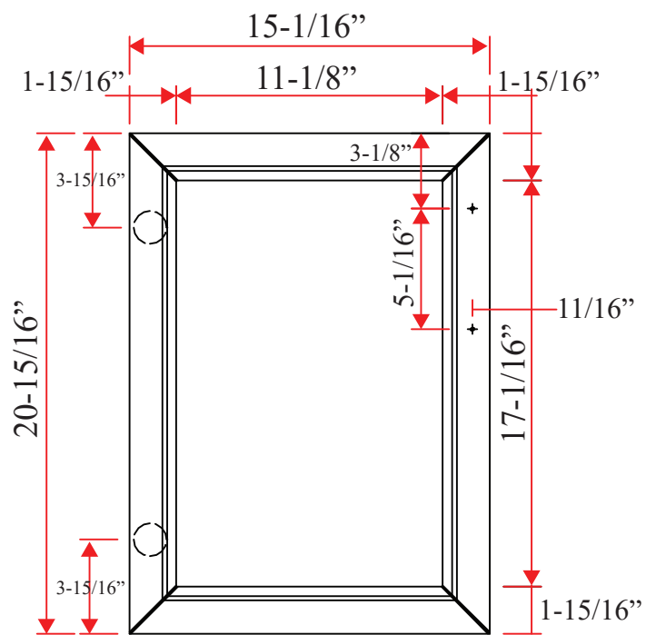
— DOOR PANEL —
