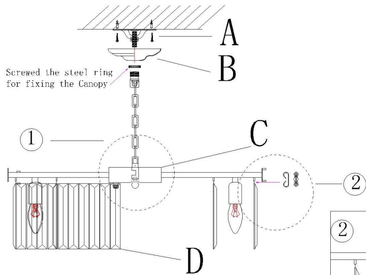
Pendant Installation
