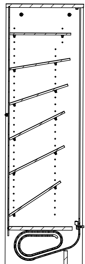
COUPE C-C ECHELLE 1 : 11
