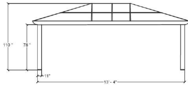
VUE DE CÔTÉ (LONGUEUR) SIDE VIEW (LENGTH)
