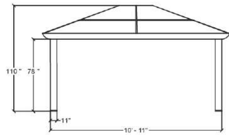
VUE DE CÔTÉ (LARGEUR) SIDE VIEW (WIDTH)
