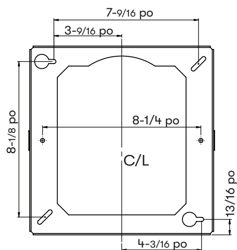
CADRE DE SUPPORT SUPÉRIEUR (vue de dessus)
