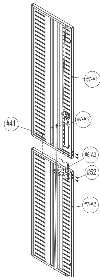
(#7-A) Right Door
