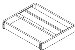
A x 2 Left armrest
