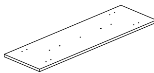
29 (1000*290*18mm x1)
