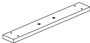
24 (500*70*18mm x2)
