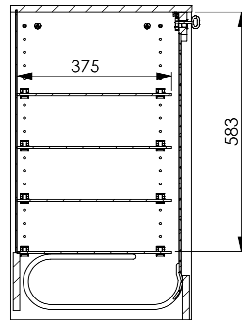
COUPE A-A ECHELLE 1 : 9
