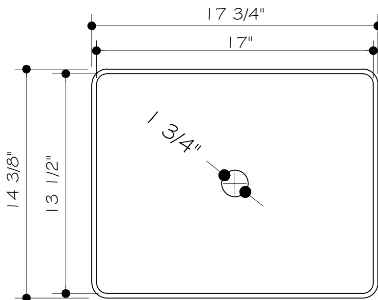
VISTA SUPERIOR
