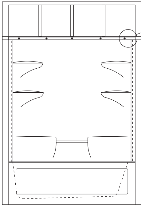
Figure 2 BA5 Fastening with Drywall Screws BA5 Fixation avec des vis pour cloisons sèches
