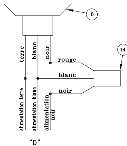
Dispositif avec Commande Photo-électrique
