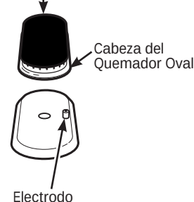
Ensamble de la Cabeza y de la Tapa del Quemador Oval (No Extraíble)
