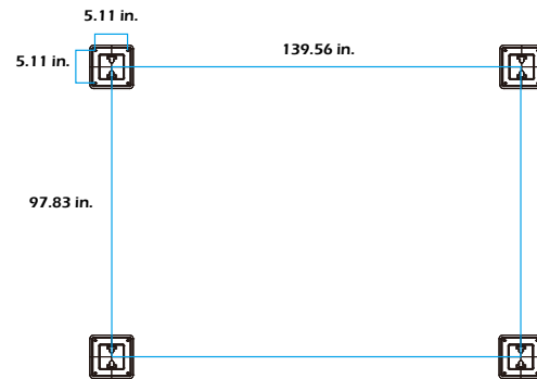
Pergola 10'x13'
