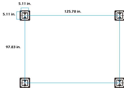
Pergola 10'x12'
