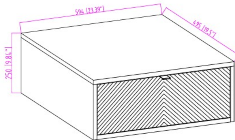
3视图
