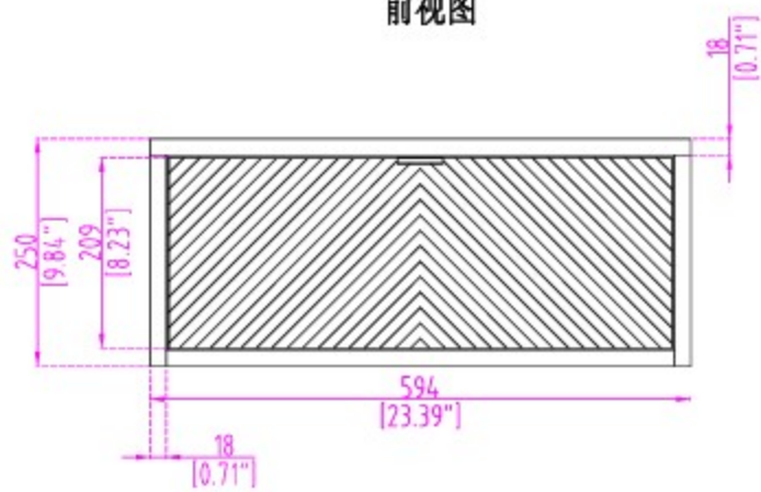
前视图
