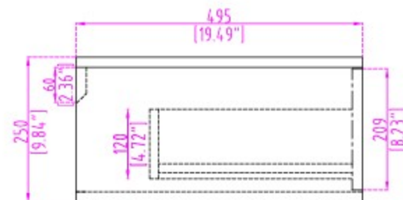
侧视图
