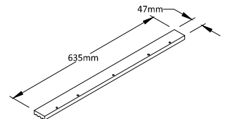
RAIL Qty:4
