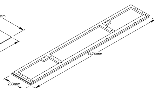
TOP Qty:1
