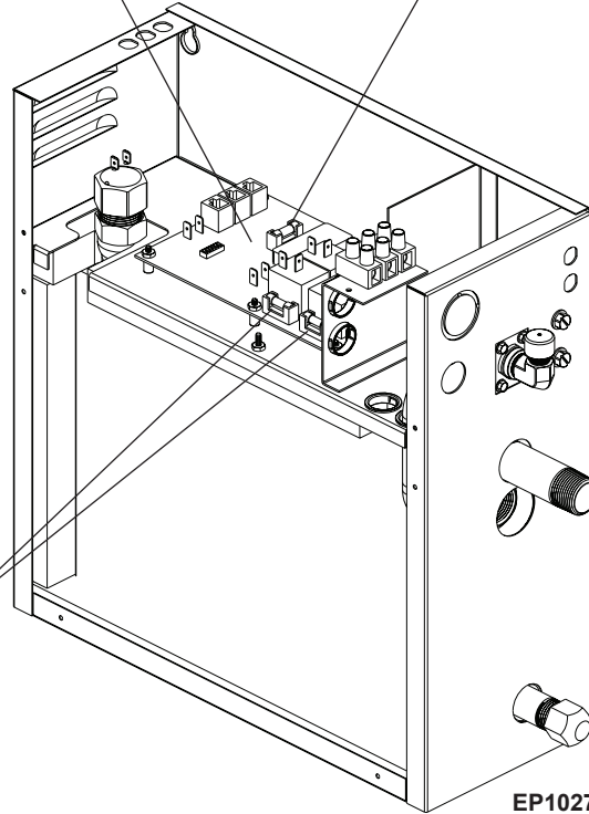
EP102738 (240V) EP102739 (208V) Auto Drain Valve Válvula de drenaje automático Électrovanne de vidange automatique
