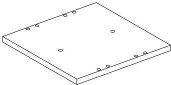
I 400*350*15mm(1pc)
