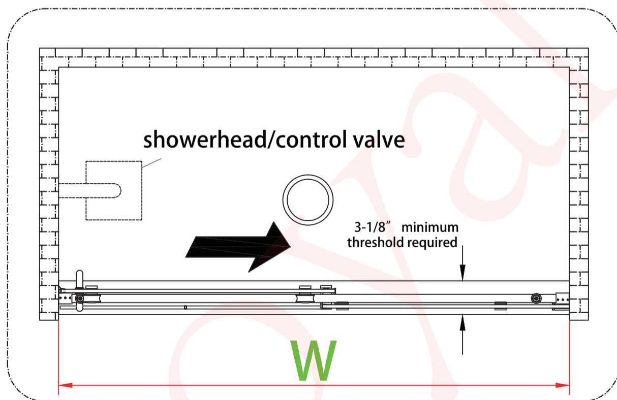
Left-hand Door
