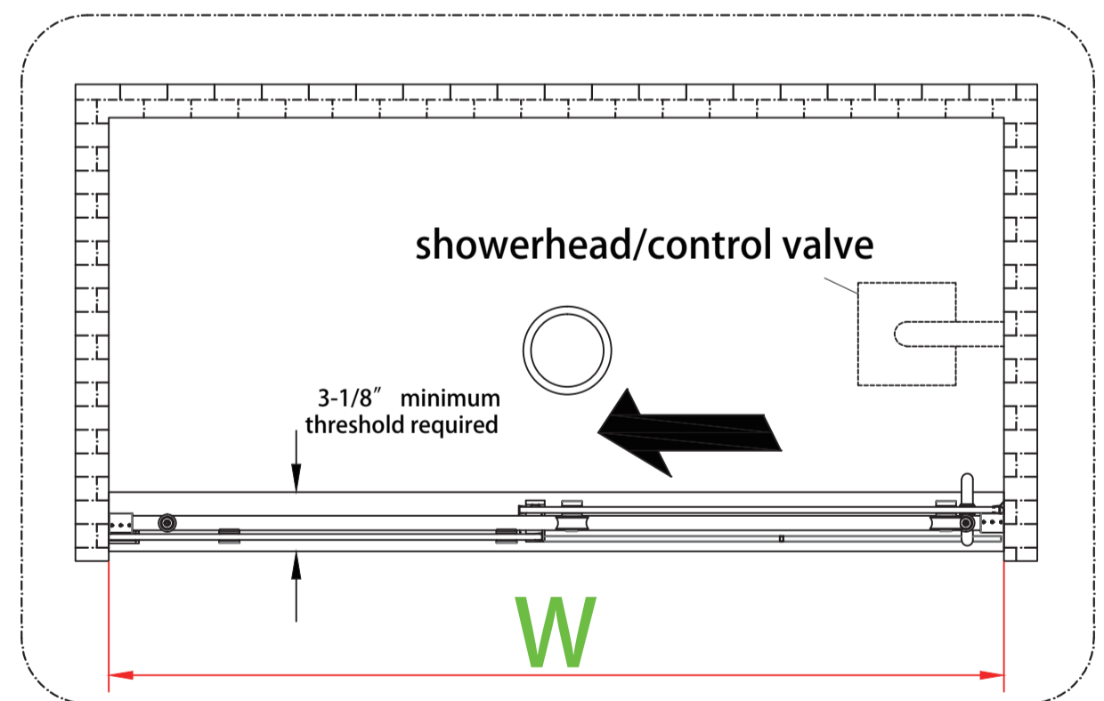
Right-hand Door
