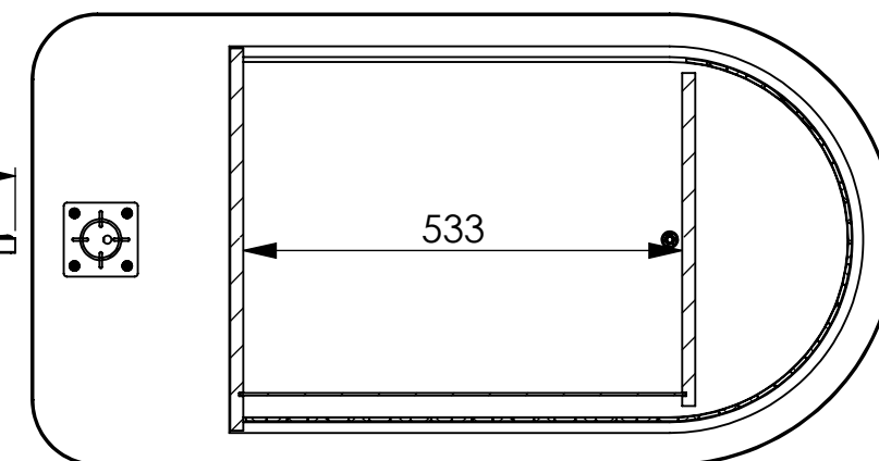
COUPE B-B
