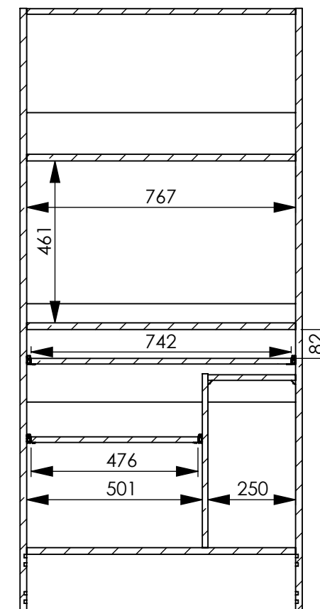
COUPE D-D ECHELLE 1 : 15.3
