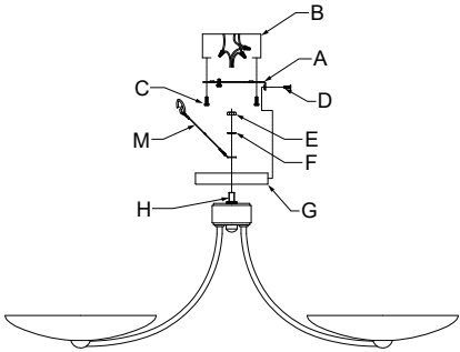
MONTAJE SEMIRRASANTE
