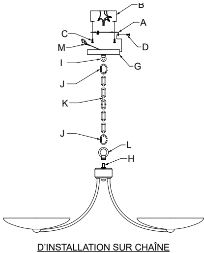
D'INSTALLATION SUR CHAÎNE
