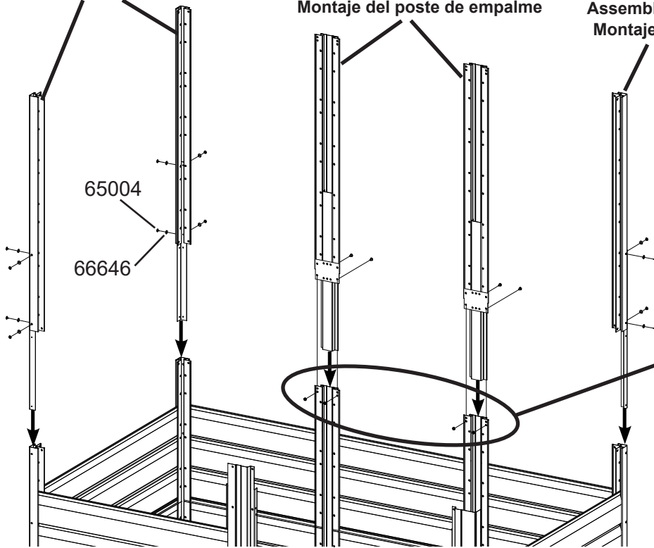
Corner Post Assembly Assemblage des poteaux d'angle Montaje del poste de la esquina
