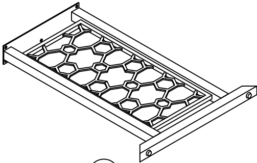
Side leg frame T4396013030KX QTY:2PCS
