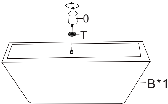
Armrest 2
