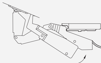
Encaje en posición
