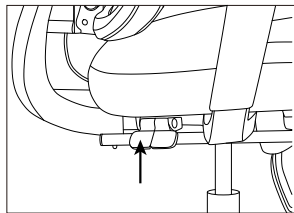
Poignée gauche : basculez pour incliner, relevez pour verrouiller.
