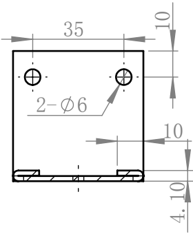
剖面 A-A
