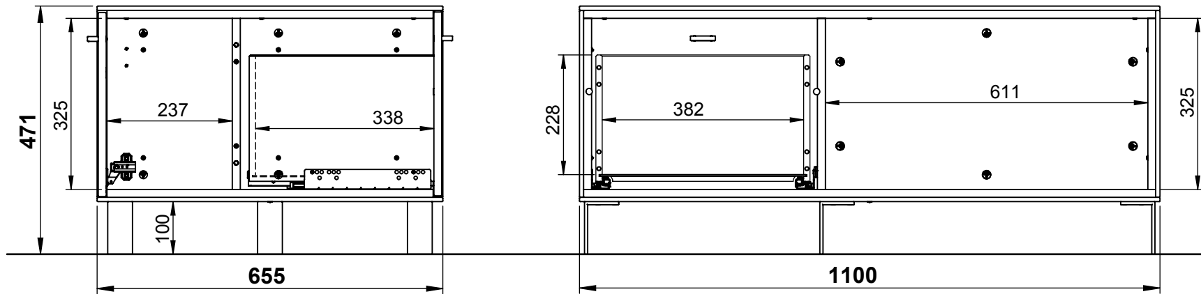
Ansicht Schubkastenseite
