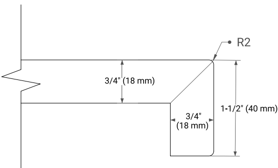
EDGE SIDE VIEW
