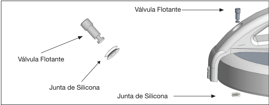
Figura: Instalación de la Válvula Flotante Inserte la valvula flotante desde la parte de arriba de la tapa y asegurela en su sitio con la goma y la parte metalica por la parte inferior de la tapa.
