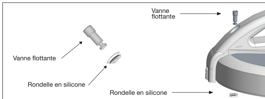
Figure : Installation de la vanne flottante
