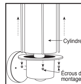
Figure 5 Appliques cylindriques
