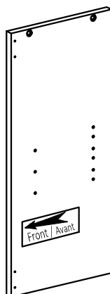
DIVIDER QTY 1
