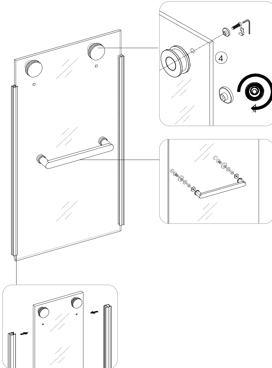
Door Glass
