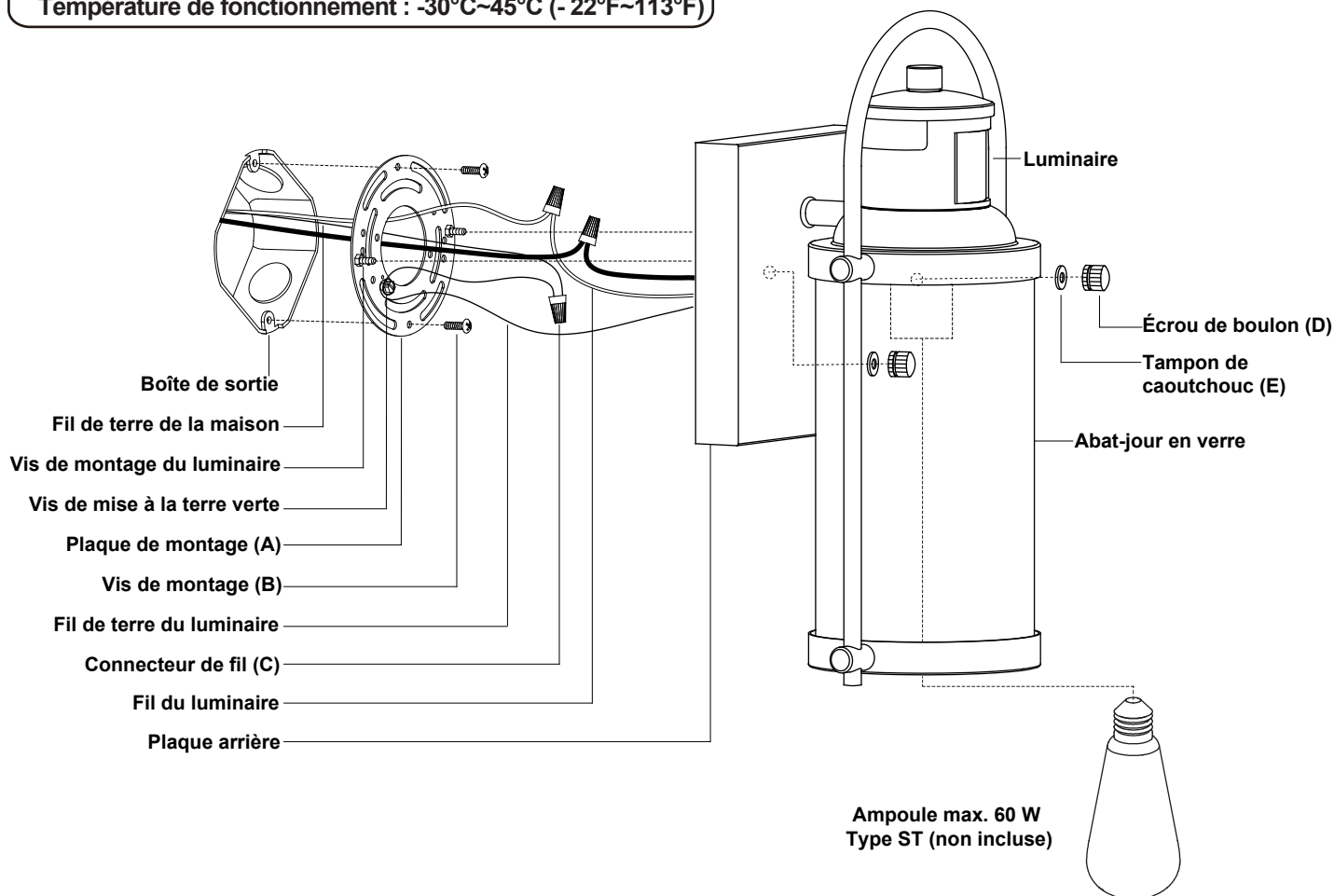
Connecteur de fil (C)
