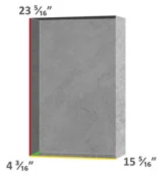
Cutout Dimensions
