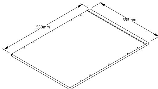
BOTTOM Qty:2
