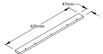
RAIL Qty:4
