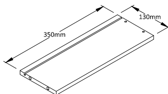
RIGHT DRAWER SIDE Qty:1
