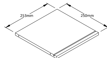
DRAWER BACK Qty:1
