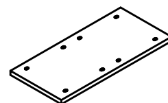
Arm connecting plates 2 pcs Plaques de connexion de bras
