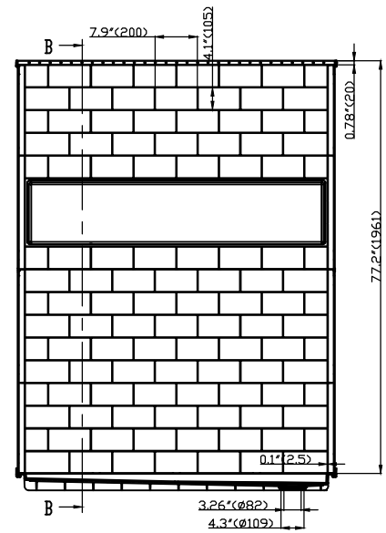
A-A
