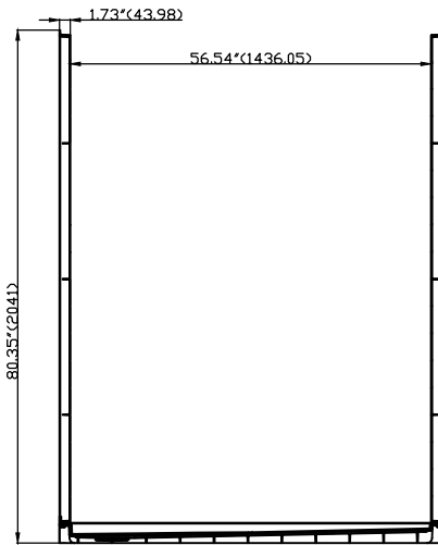
D-D
