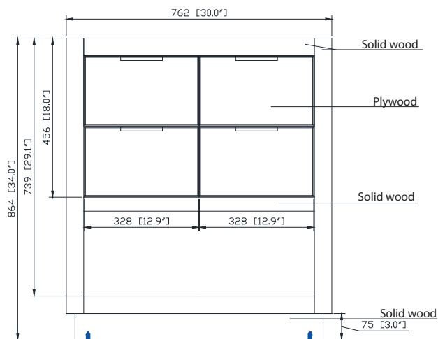
Front / Devant
