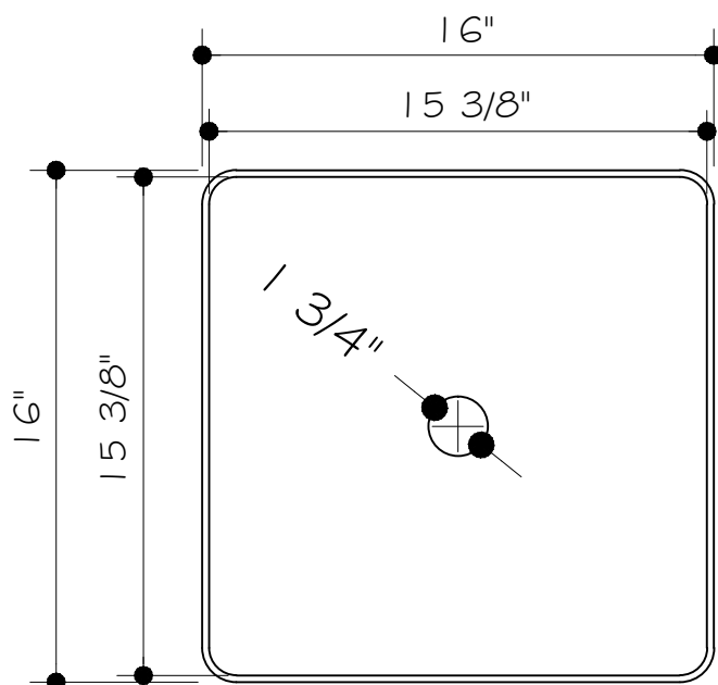
VISTA SUPERIOR
