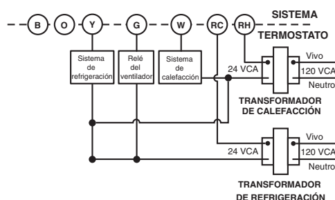
Figura 5. Diagrama de conexiones típico para sistemas de calor/frío de dos transformadores y 5 cables
