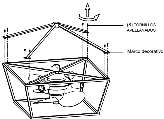
Plano de desmontaje del marco decorativo
