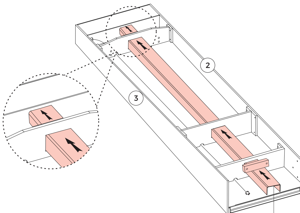
FIG. 5 Assembly / Montaje FIG. 5 / FIG. 5 Assemblage
