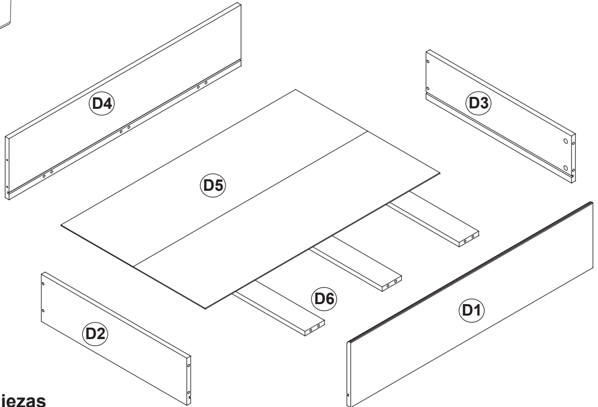
Left Drawer Side (2) Côté gauche du tiroir Lado del cajón izquierdo
