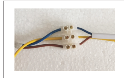
6.驱动器输入电源线与家用电源线用接线端子对接好，锁紧螺丝即可。
