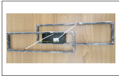
3.第二个灯框错开组装在底盘上，地线任意套在其中一款螺丝上。
