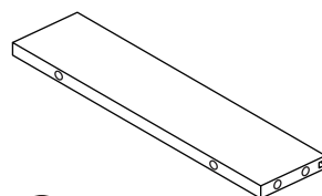
G 400*100*12mm(2pcs)
