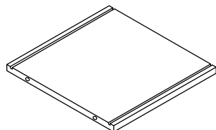
L 298*285*12mm(1pc)
